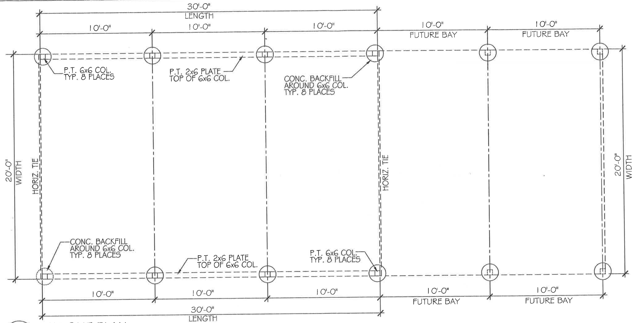
1 LAY-OUT PLAN A1 1/4" = 1'-0"
